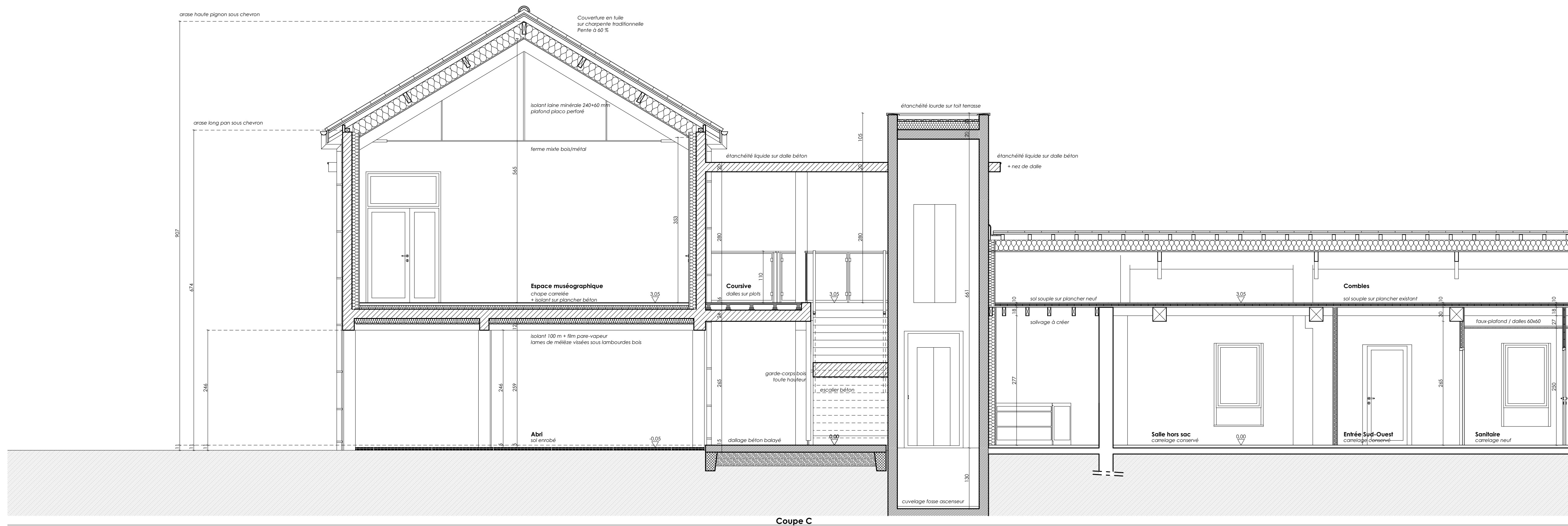
Coupe C
