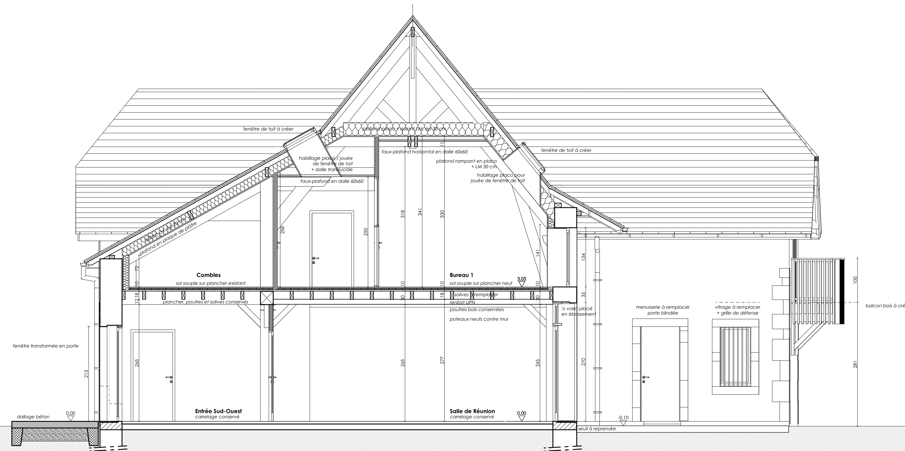
Coupe 1
