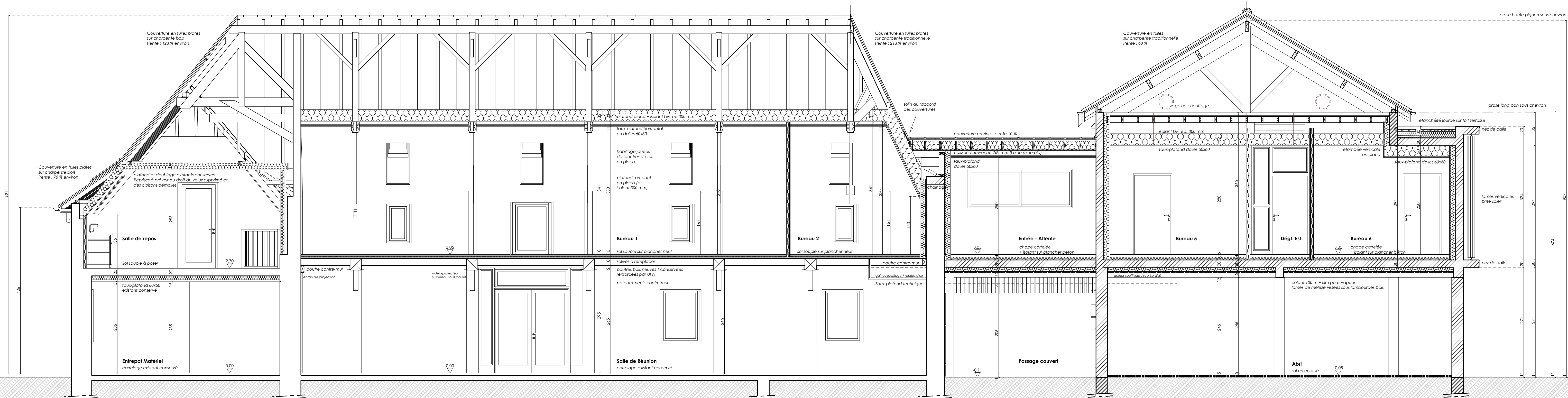
Coupe A
